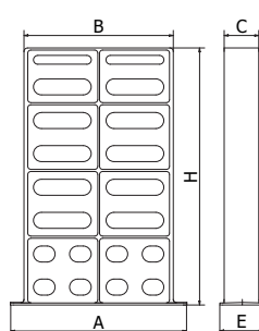
WZP/2D/6/5/6 DŁ. 320 NAT
